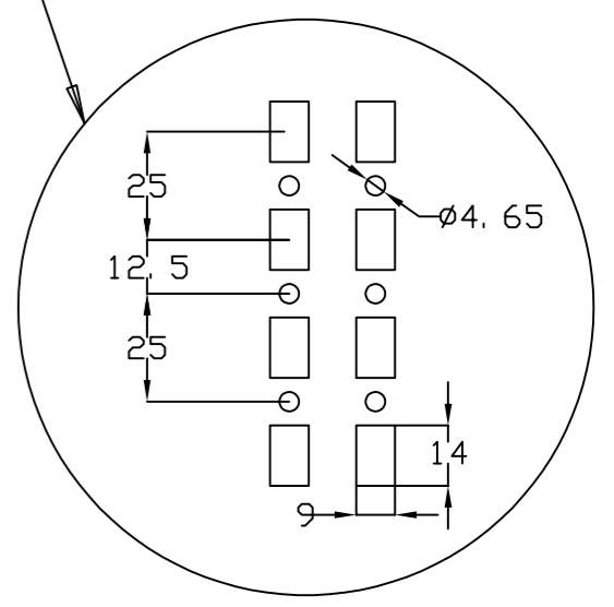
DETALLE DEL PERFIL PROFILE DETAIL
