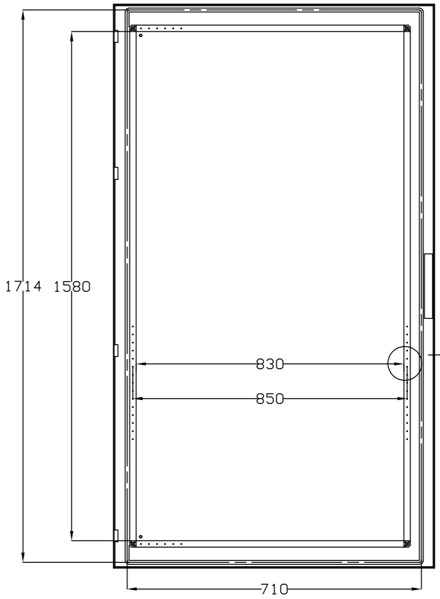
VISTA POSTERIOR PUERTA DOOR REAR VIEW
