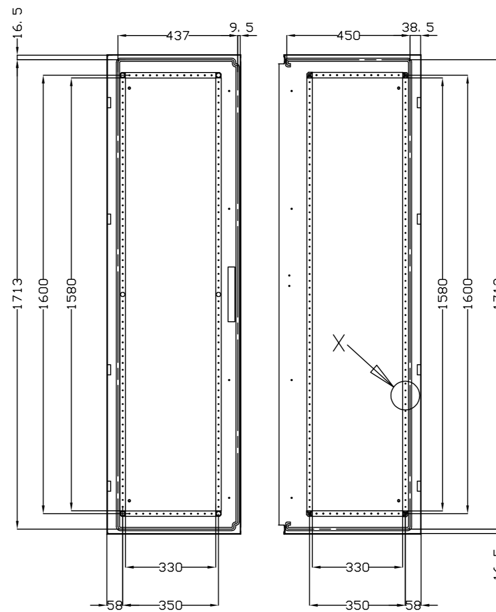
VISTA POSTERIOR PUERTA DOOR REAR VIEW
