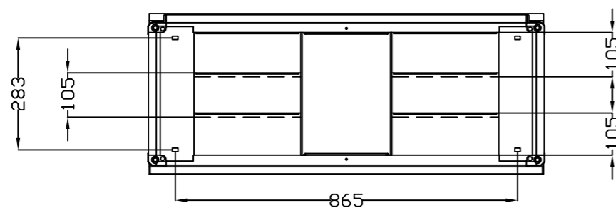
VISTA INFERIOR BOTTOM VIEW
