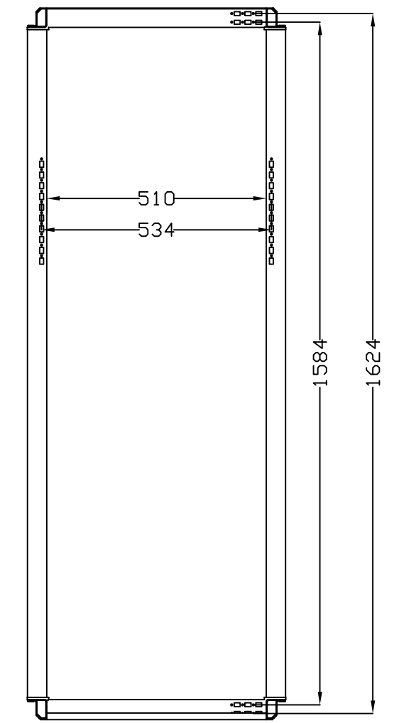
SEC. A-A
