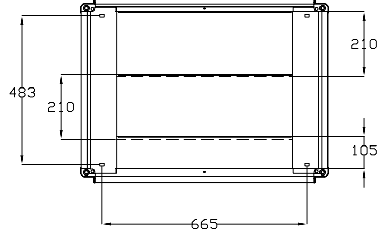
VISTA INFERIOR BOTTOM VIEW
