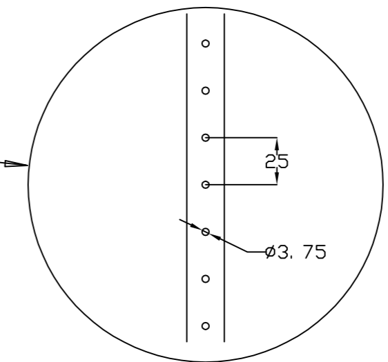
DETALLE DEL REFUERZO PROFILE DETAIL
