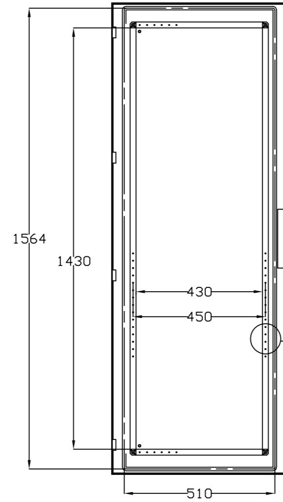
VISTA POSTERIOR PUERTA DOOR REAR VIEW
