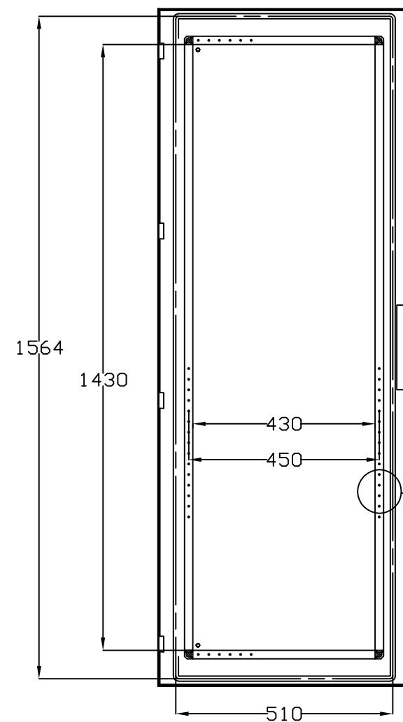
VISTA POSTERIOR PUERTA DOOR REAR VIEW
