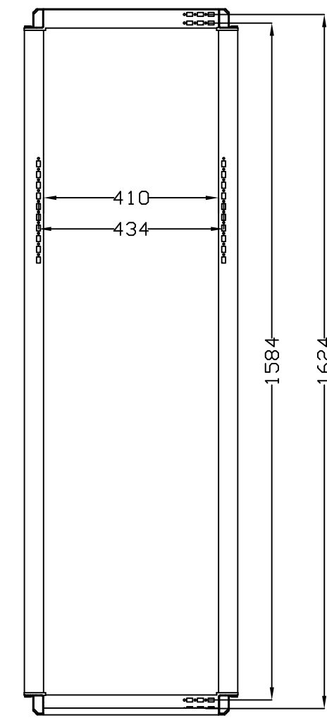
SEC. A-A
