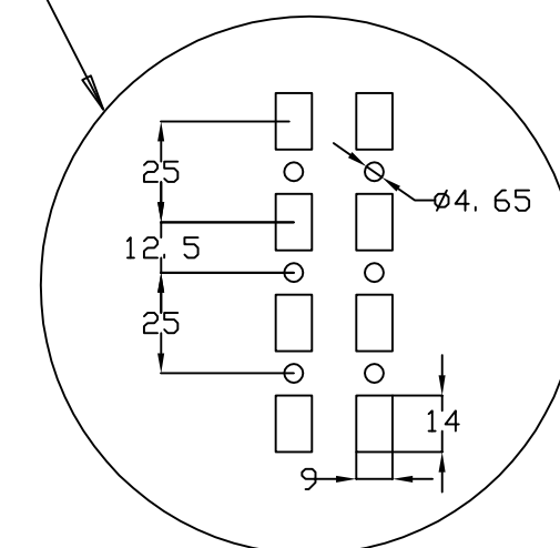
DETALLE DEL PERFIL PROFILE DETAIL
