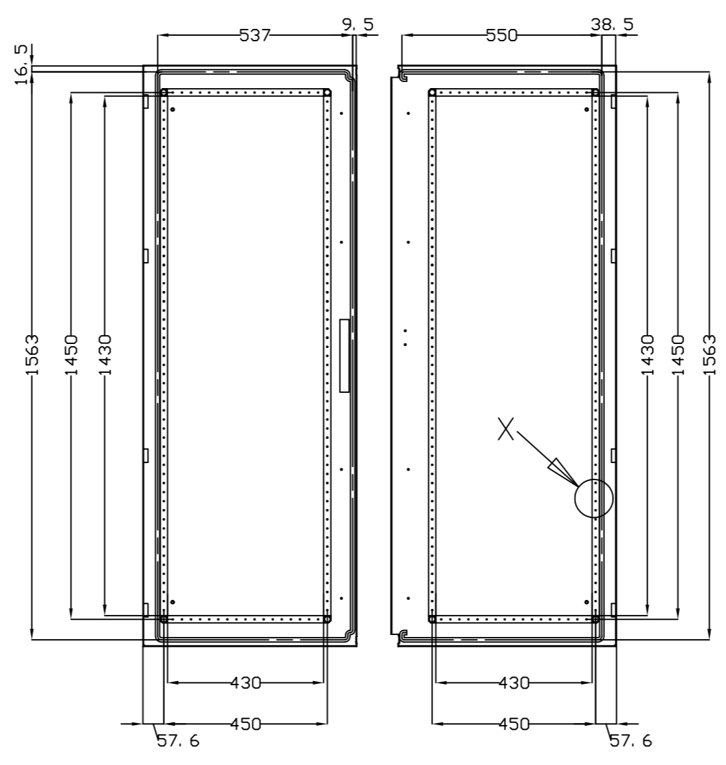
VISTA POSTERIOR PUERTA DOOR REAR VIEW
