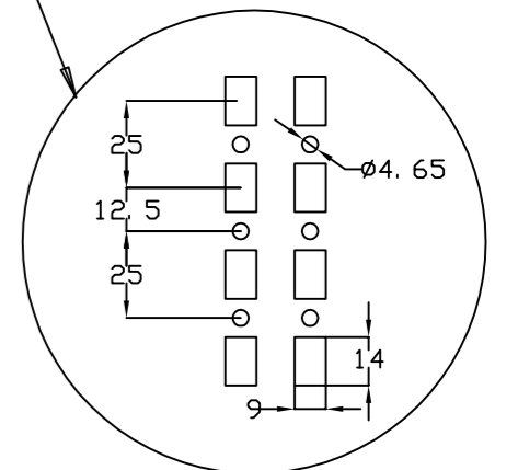
DETALLE DEL PERFIL PROFILE DETAIL
