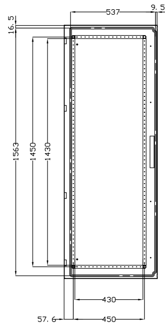
VISTA POSTERIOR PUERTA DOOR REAR VIEW
