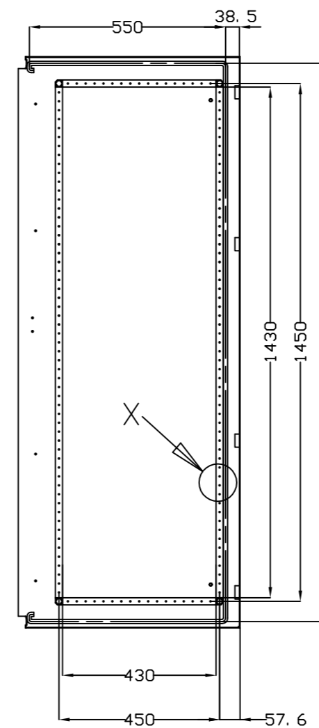
VISTA POSTERIOR PUERTA DOOR REAR VIEW
