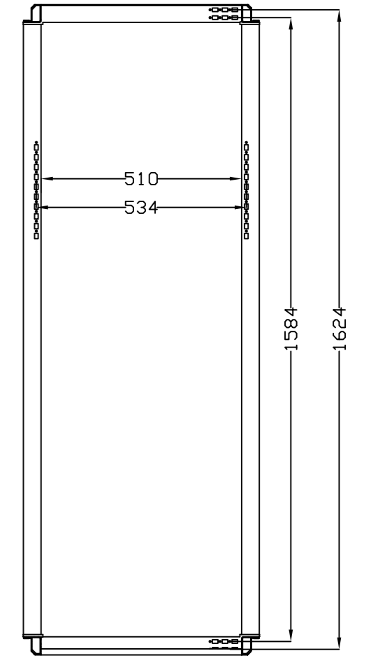
SEC. A-A
