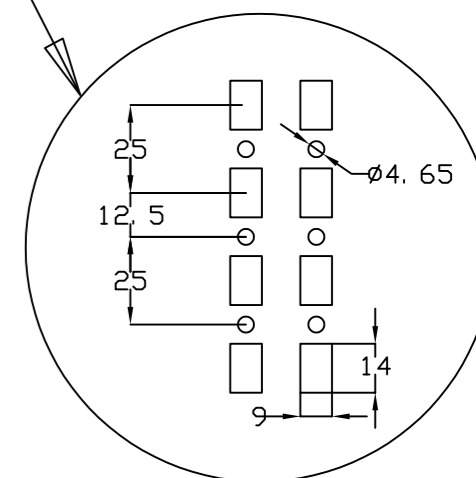
DETALLE DEL PERFIL PROFILE DETAIL
