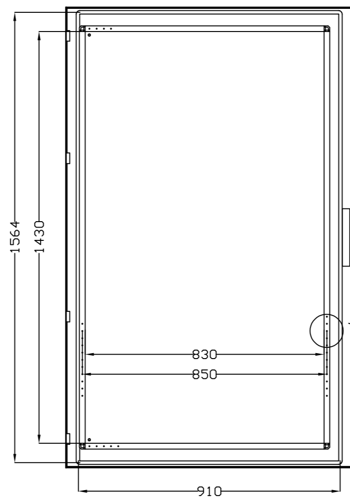
VISTA POSTERIOR PUERTA DOOR REAR VIEW
