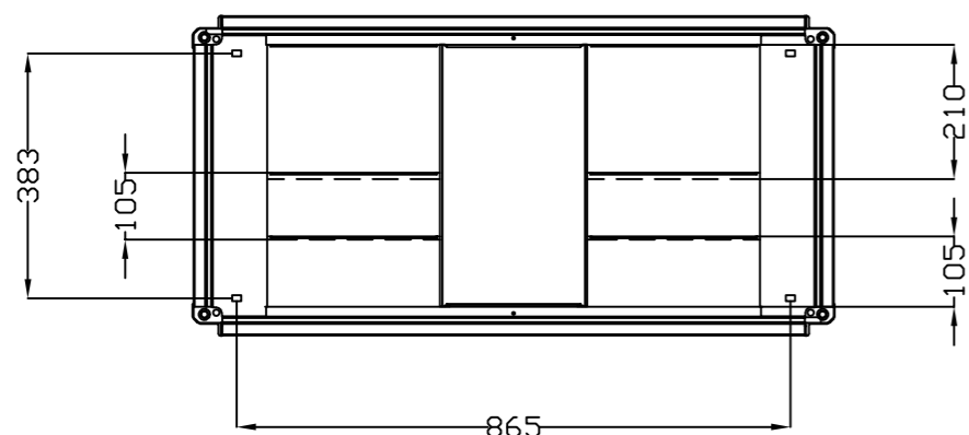
VISTA INFERIOR BOTTOM VIEW
