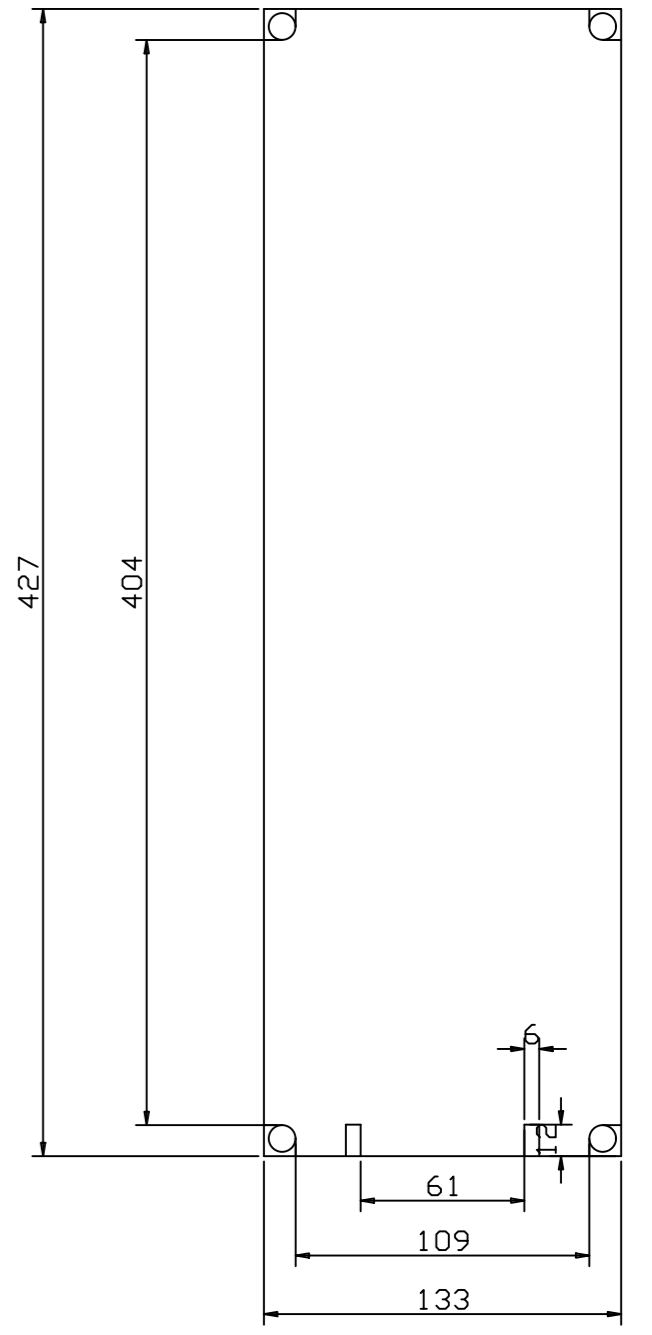
DETALLE ZONA UTIL DE TRABAJO/ DETAIL OF WORKING AREA
