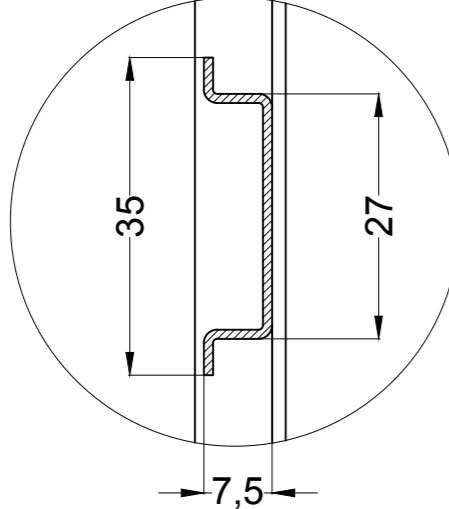
DETALLE A
