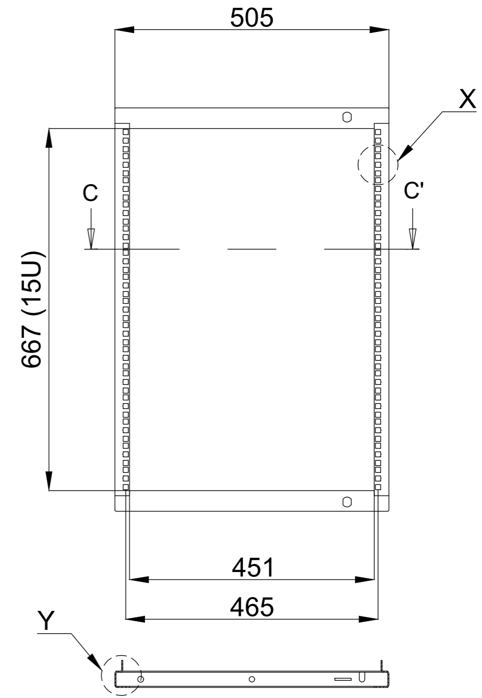
CORTE C-C'
