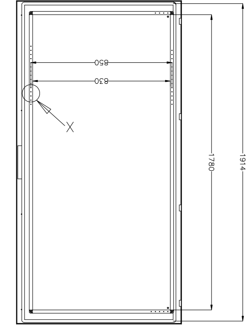
VISTA POSTERIOR PUERTA DOOR REAR VIEW
