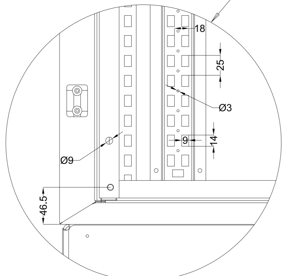
DETALLE DEL PERFIL PROFILE DETAIL
