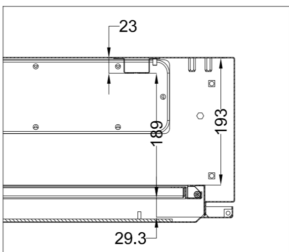
TAPA MODULAR/CIEGA MODULAR/BLIND LID
