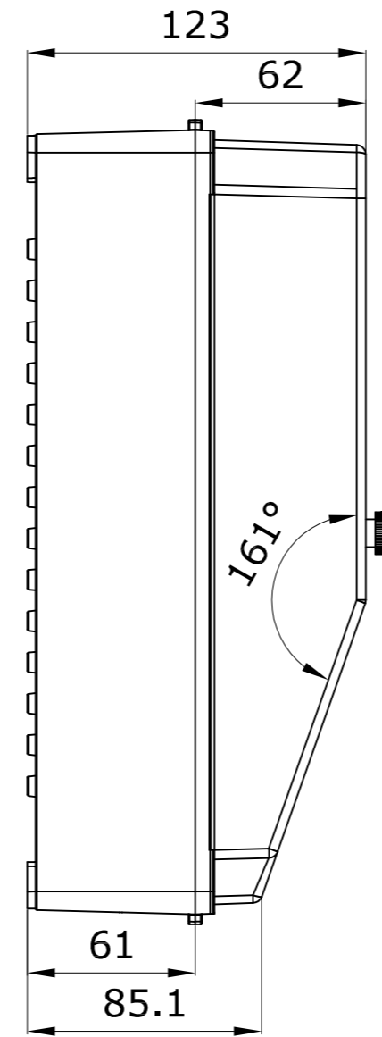
DETALLE ZONA UTIL DE TRABAJO/ DETAIL OF WORKING AREA 204
