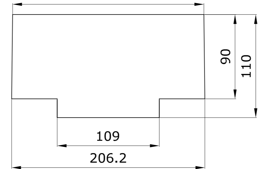
DETALLE ZONA UTIL DE TRABAJO/ DETAIL OF WORKING AREA 204
