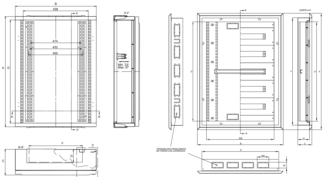
DETALLE DE SECCIÓN (Z) ARMARIO ENLAZABLE
