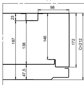
DETALLE DE SECCIÓN (Z) SUPERFICIE IP40
