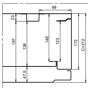
DETALLE DE SECCIÓN (Z) ARMARIO ENLAZABLE
