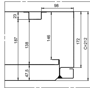
DETALLE DE SECCIÓN (Z) SUPERFICIE IP65
